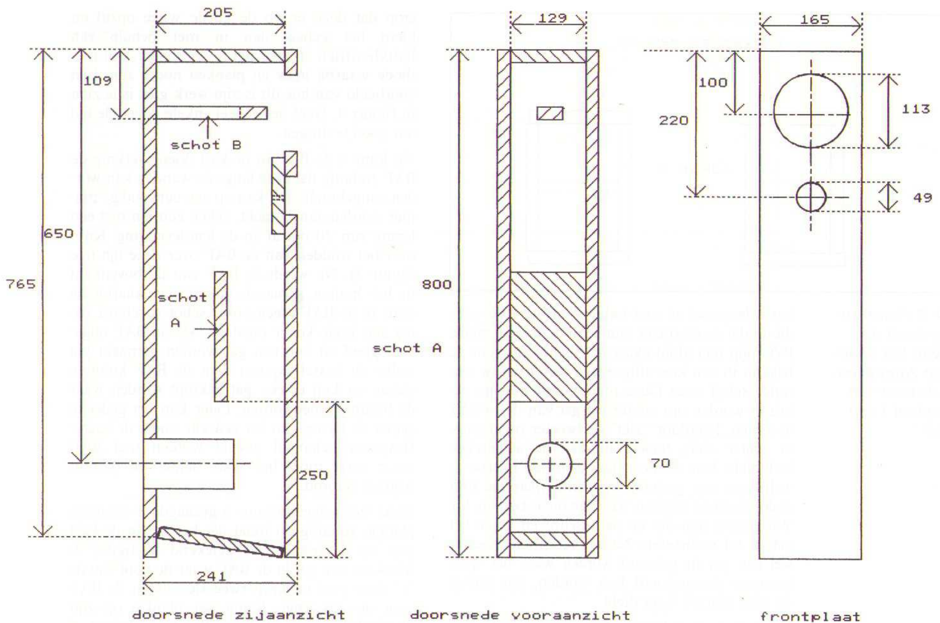
Figuur 2. De constructie van 'Freek'.
